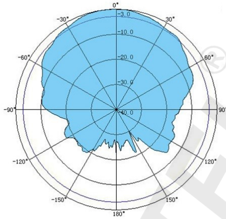
ГОРИЗОНТАЛЬНАЯ ПЛОСКОСТЬ
